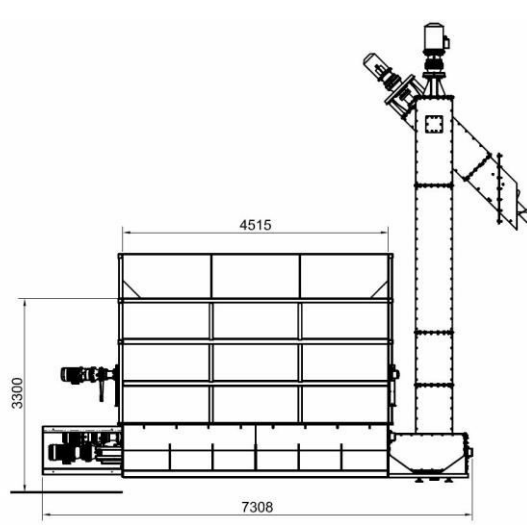
Seitenansicht
