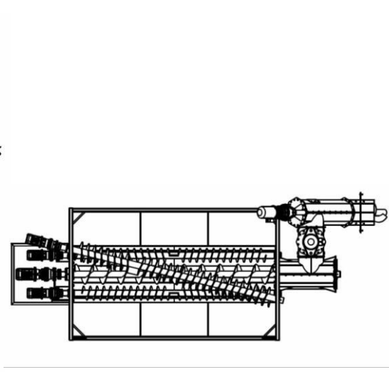
Draufsicht
