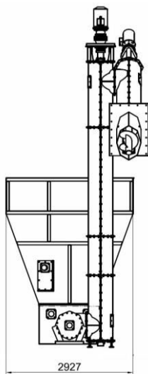
Frontansicht
